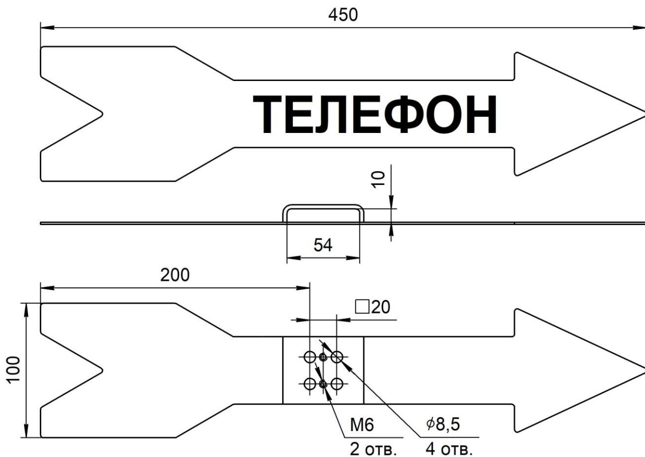
Указатель-стрелка "ТЕЛЕФОН" правый БРМТ.305442.002
