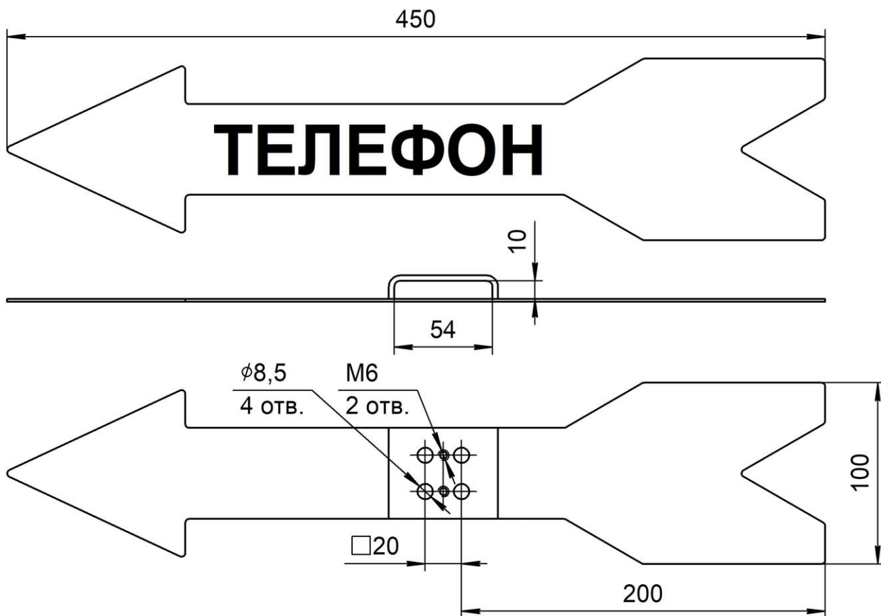
Указатель-стрелка "ТЕЛЕФОН" левый БРМТ.305442.002
