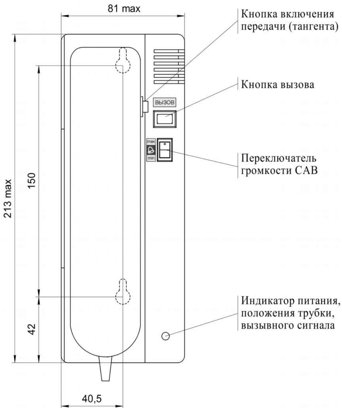
Рисунок 1 - Габаритные размеры и назначение органов управления и индикации АТ-П-02М1
