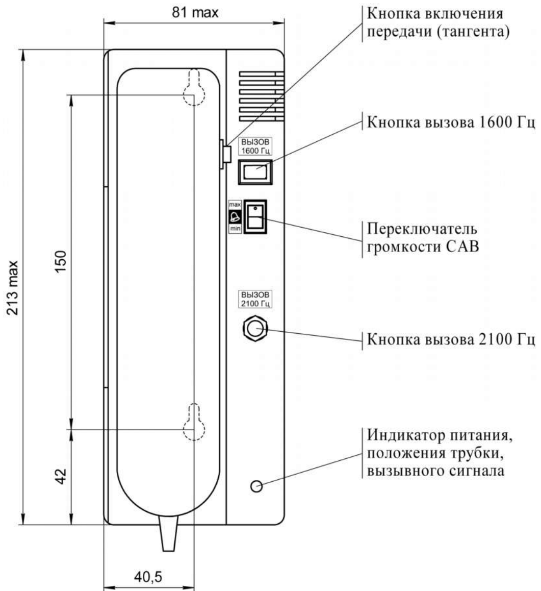
Рисунок 1 - Габаритные размеры и назначение органов управления и индикации АТ-П-02М2
